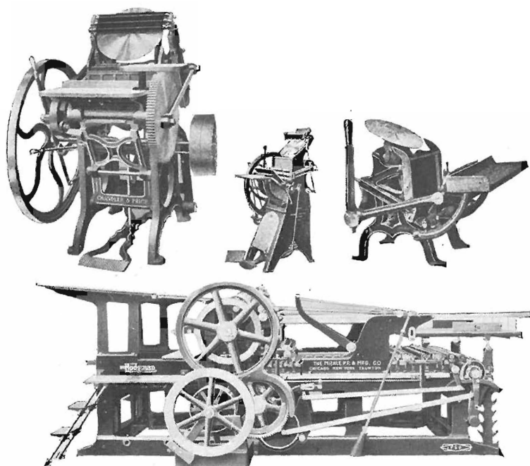
Osa Suom. Sos. Kustannusyhtiön painokoneistoa.
