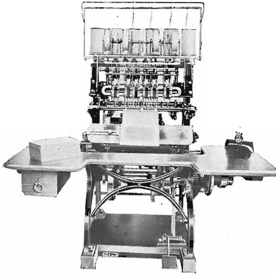
Sitomo-ompeelukone.
