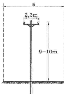
Paljas avajohto
