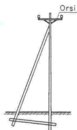
A-kulmapylväs
