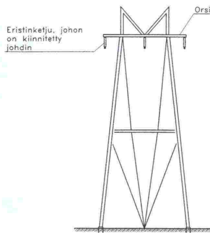
Harustettu portaalipylväs
